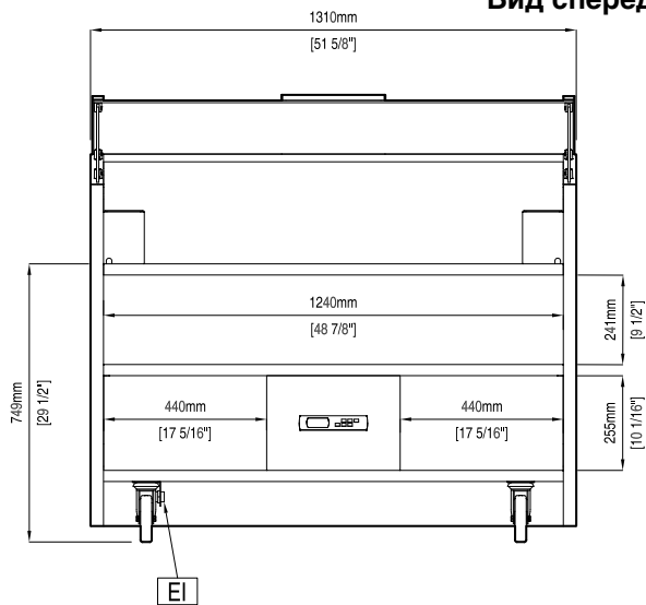
Вид сбоку
